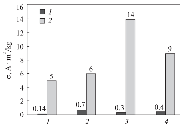
Рис. 2. Значення намагніченості насичення зразків до (1) та після перетворення (2): 1 — гетитова руда Керченського залізорудного басейну (зр. 1); 2 — гетитова руда Криворізького залізорудного басейну (зр. 2); 3 — гематитовий концентрат, отриманий з гематитової руди Криворізького залізорудного басейну (зр. 3); 4 — гематитова руда Криворізького залізорудного басейну (зр. 4)
