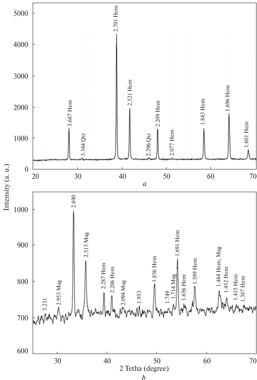
Рис. 3. Дифрактограма вихідного ( a - \text{CoK}_\alpha ) та перетвореного ( b - \text{CuK}_\alpha ) зразка гематитового концентрату, отриманого з гематитової руди Криворізького залізорудного басейну
