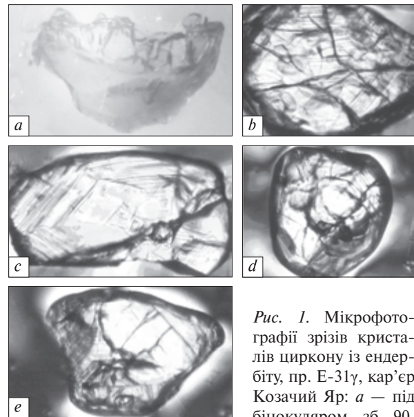
Рис. 1. Мікрофотографії зрізів кристалів циркону із ендербіту, пр. E-31γ, кар'єр Козачий Яр: а — під бінокулярним зб. 90, б—е — під поляризаційним мікроскопом, Нік. +, зб. 240
