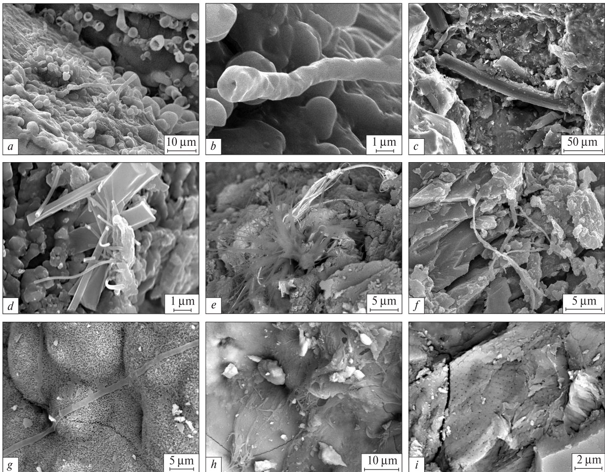
Рис. 7. Видовжений тип продуктів вивітрювання в метеоритах: a — асоціація об'єктів трубчастої, сталактитоподібної і циліндричної форм із мікросфероїдами; b, c — відповідно, закриті і порожнисте трубчасті утворення; d — агрегат видовжених евгедральних та деформованих ниткоподібних кристалів рабдиту (?) в корозійній кірці по зерну ОІ, паласит Брагін; e–g — нитко- і ламелеподібні утворення; h, i — неідентифіковані об'єкти складної форми: h — дендритоподібний, i — шаруватий з регулярно розташованими порами. Відколи хондритів Кулішівка ( a ), Біла Церква ( b, c ), Грузьке ( e–i )
