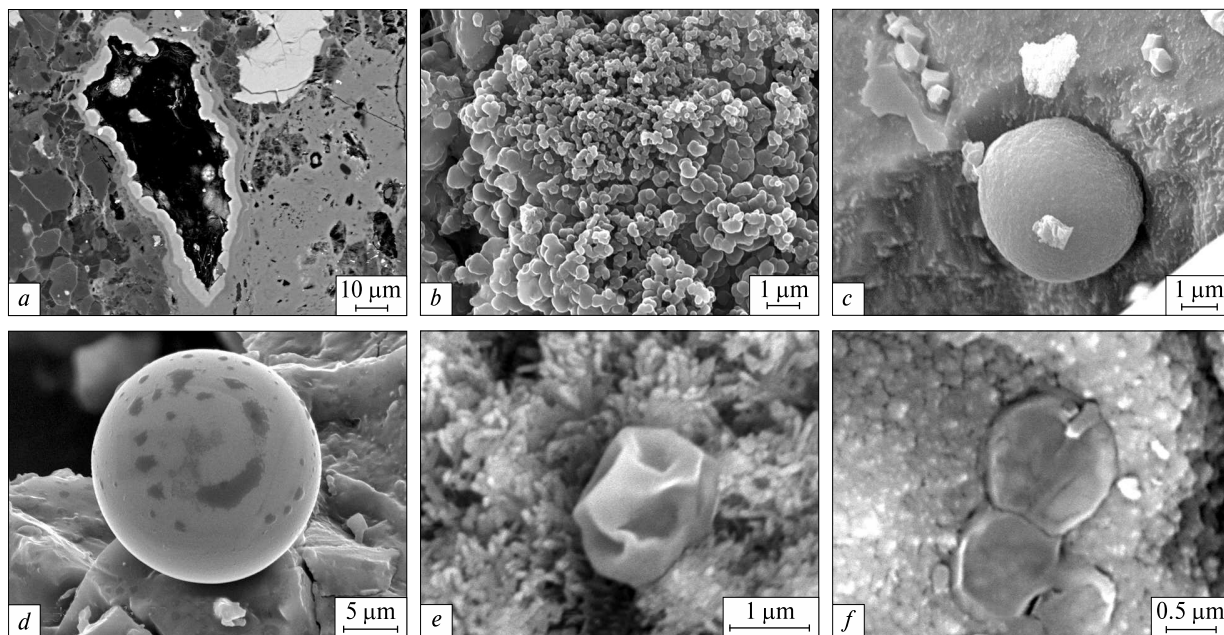
Рис. 5. Ізометричні утворення на поверхні вивітрених зразків метеоритів: a — мікросекреція лінозоподібної форми в силікатній матриці, на стінках якої утворились напівсфероїди зональної будови і кульки мікроглобулярної будови, хондрит Грузьке, полірований шліф; b — мікроглобулярні агрегати гідроксидів Fe у заглибленні на поверхні металеві пластинки з атакситу Чінге, на якій відсутні кулясті утворення. Щільні кульки: c — в асоціації з ізометричними субмікриметровими кристалами на поверхні зерна нікелістого заліза, відкол хондрита Біла Церква, d — на поверхні відколу хондрита Жовтневий Хутір; e — мікроспора. f — нез'ясовані біологічні об'єкти, відкол хондрита Грузьке
