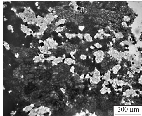
Рис. 5. Асоціація пізньої генерації аланіту (темний) з епідотом (світлий). Обидва мінерали з характерними тріщинами усихання Fig. 5. Association of later generation of allanite (dark) with epidote (light). Both minerals have characteristic shrinkage cracks
