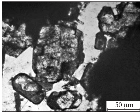
Рис. 3. Ізометричні кристали епідоту в зальбандах кварцової мигдалини Fig. 3. Isometric epidote crystals in quartz amygdaloidal selvage
