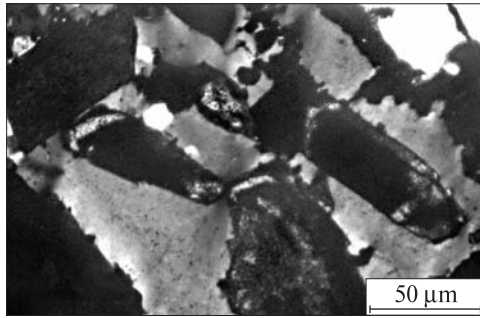
Рис. 2. Зонально забарвлені двоголові кристали аланіту в зальбандах кварцової мигдалини. Ніколі + Fig. 2. Zonal colored bi-tops allanite crystals in quartz amygdaloidal selvage. Nicole +
