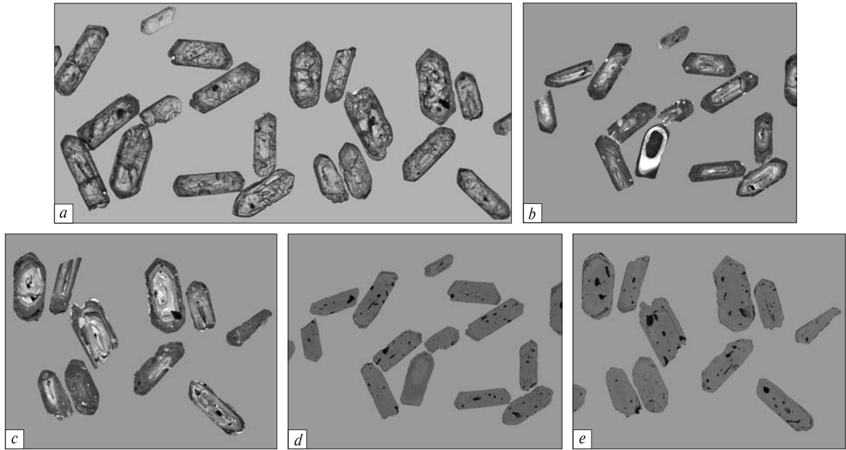
Рис. 7. Кристали циркону із рівномірнозернистого граніту (пр. КД-2): a — поляризаційний мікроскоп, наскрізне світло, ніколи паралельні, зб. 200; b–e — растровий електронний мікроскоп; b, c — катодолумінесценція; d, e — режим BSE
