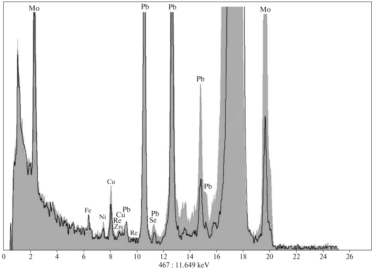
Рис. 5. Спектр характеристичного рентгенівського випромінювання кристала пержанського молібденіту Fig. 5. The characteristic X-ray spectrum of the Percha molybdenite crystal
